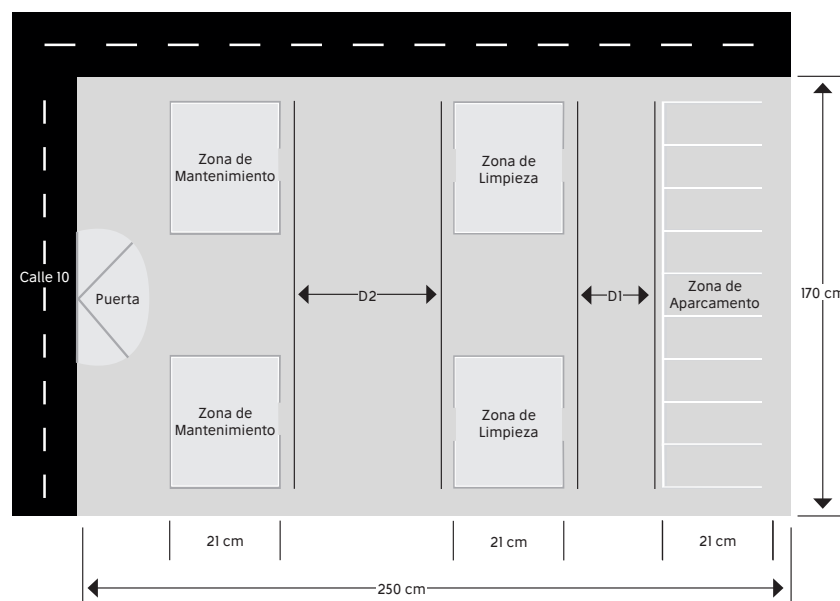
Figura 2. Plano del centro de Acopio. Elaboración propia
