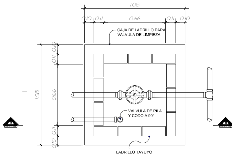
PLANTA VALVULA DE PURGA
