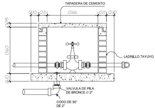
CORTE B-B VALVULA DE PURGA
