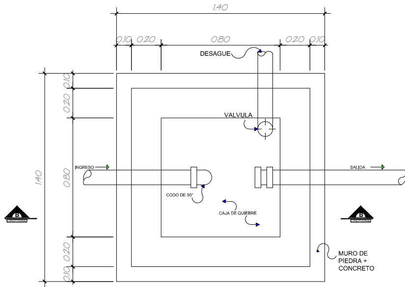
PLANTA CAMARA DE QUIEBRE
