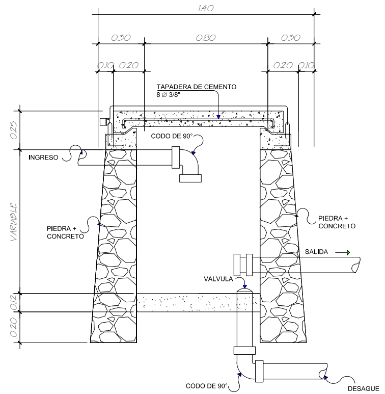
CORTE B-B CAMARA DE QUIEBRE
