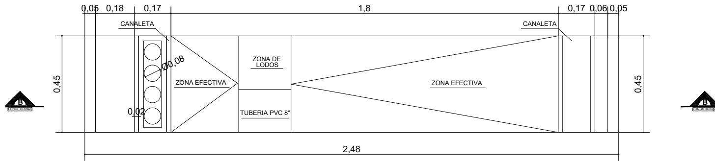
PLANTA DESARENADOR ESCALA 1:1
