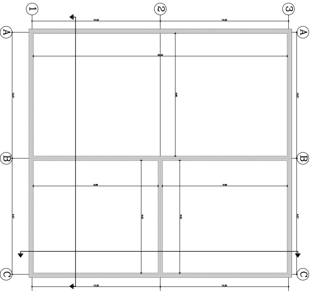
PLANTA ESTRUCTURAL MUROS
