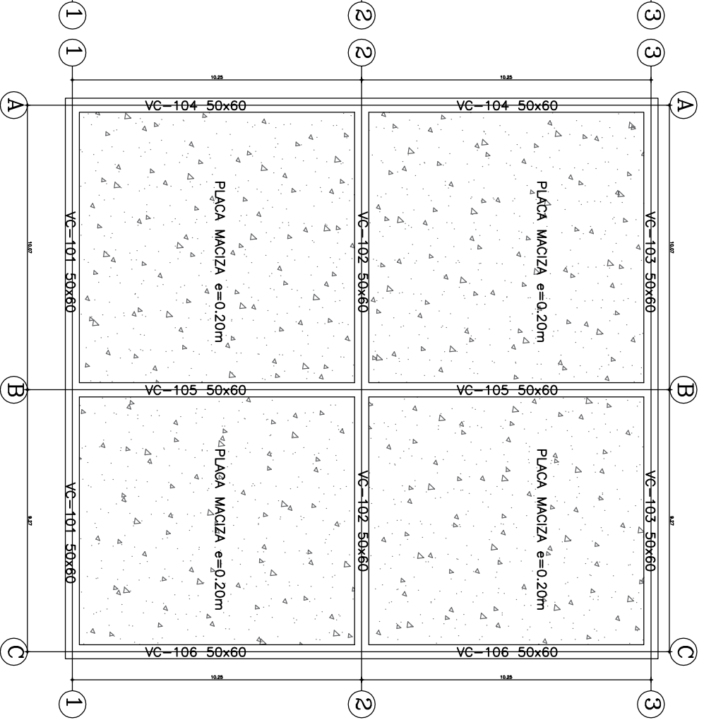
PLANTA DE CIMENTACION
