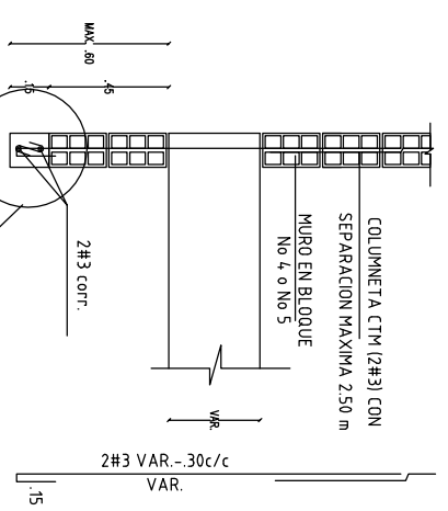
DETALLE DE DINTEL ESC: 1:25
