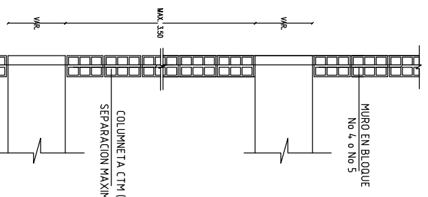
CORTE 1-1 ESC: 1:25
