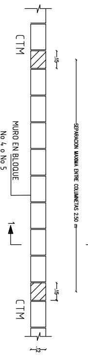
DETALLE VISTA EN PLANTA MURO FACHADA CONFINADO ESC: 1:25
