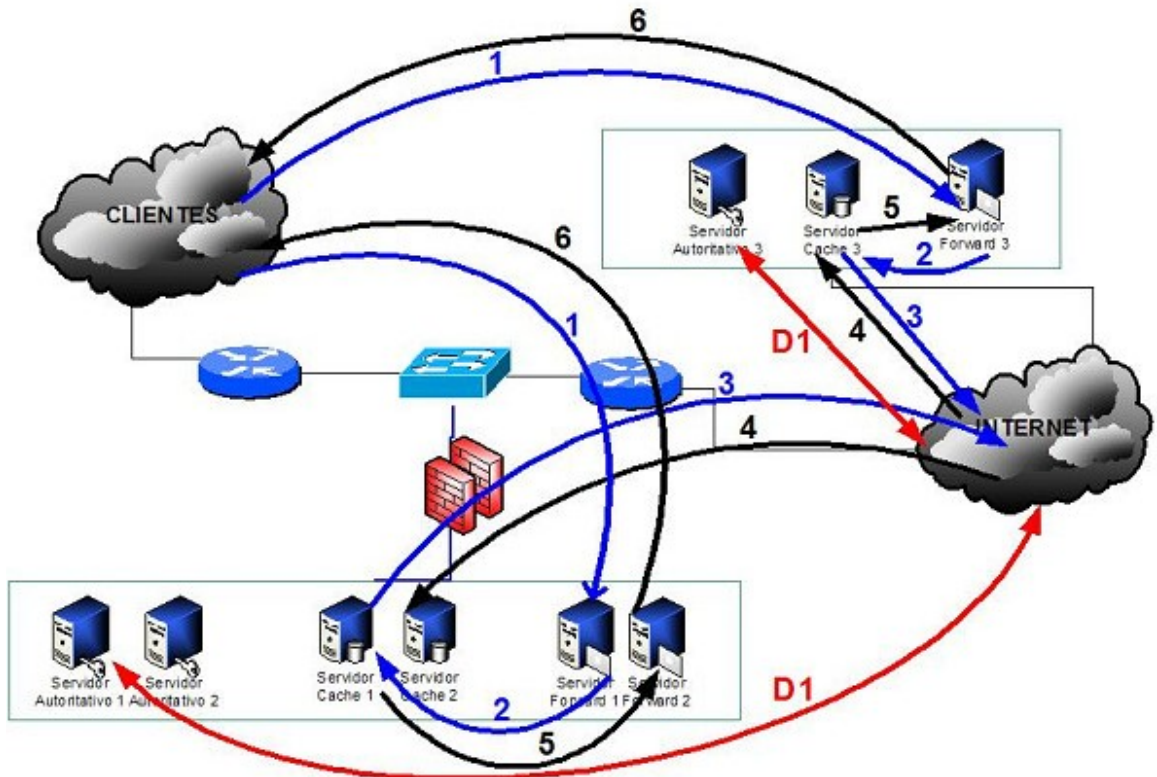
Figura 1. Arquitectura DNS
