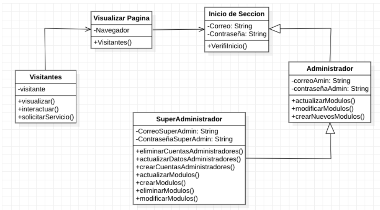
Figura 25. Diagrama De Clase
