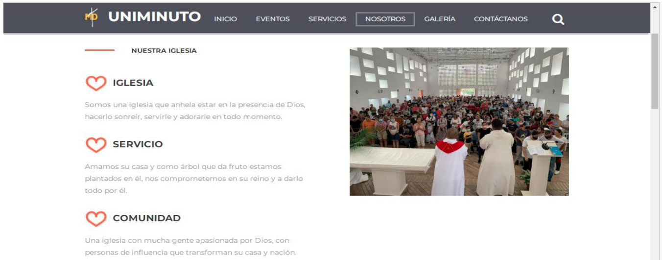
Figura 44. Sección Nosotros
