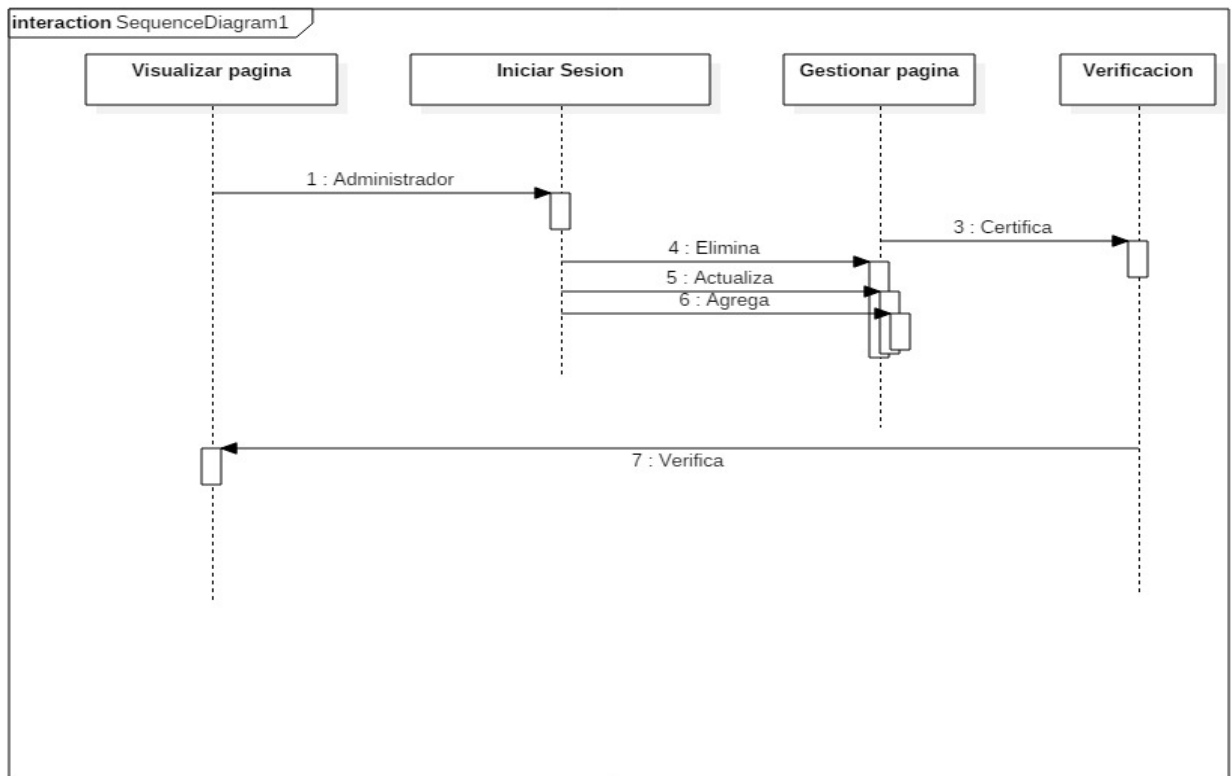
Figura 9. Diagrama De Secuencia
