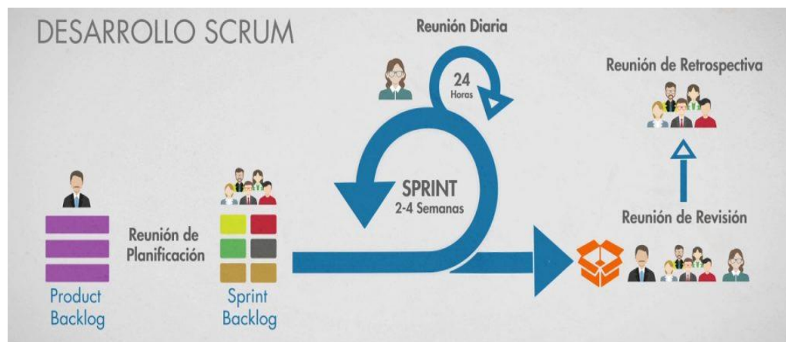
Figura 6. Metodología Scrum
