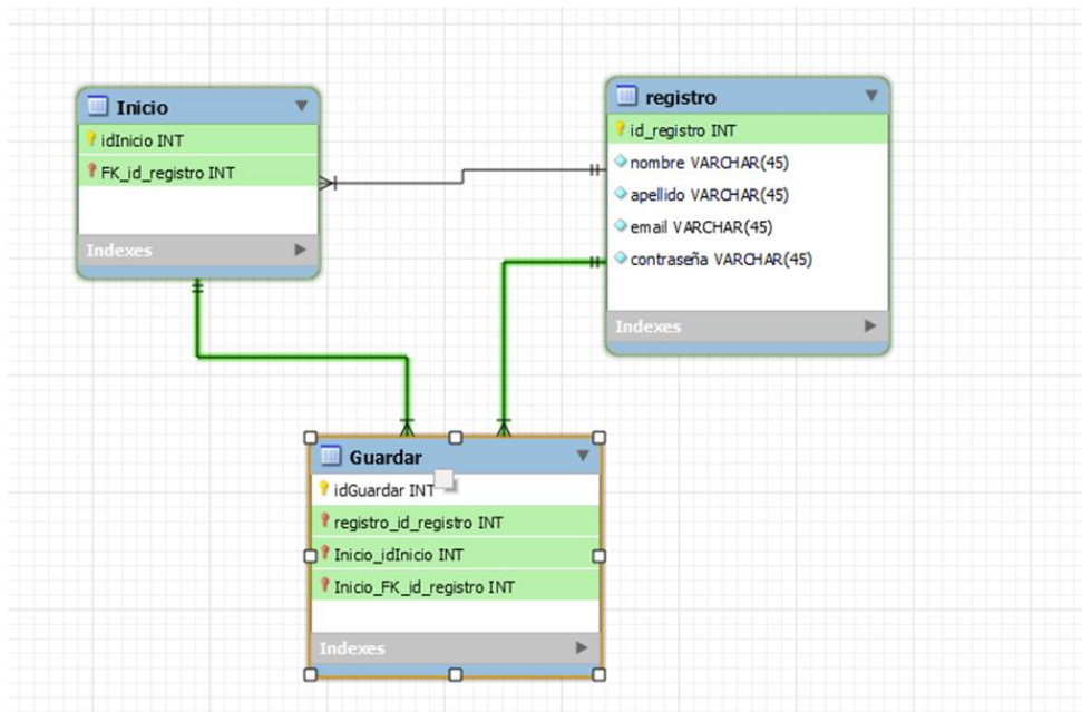
Figura 4. Modelo relacional
