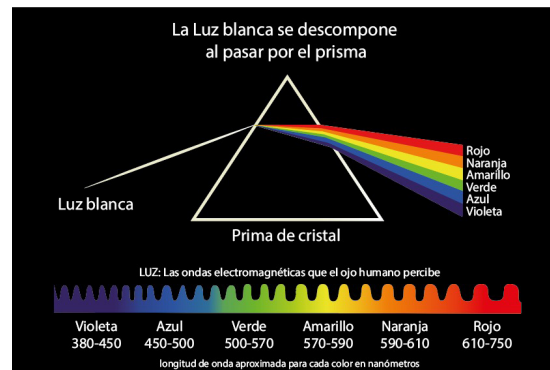
Figura 1. Espectro visible. Elaboración propia
