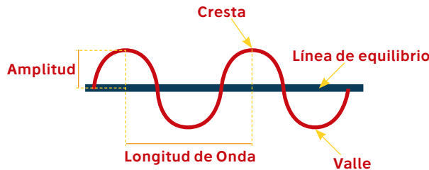
Figura 4. Longitud de onda. Elaboración propia
