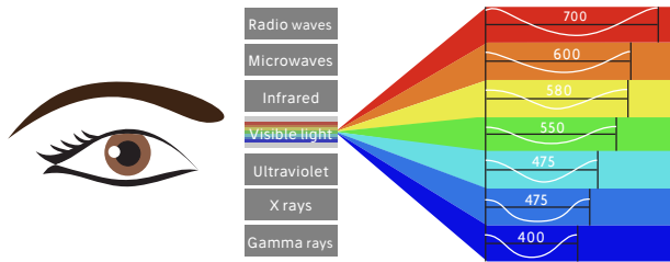
Figura 3. Luz visible. Elaboración propia
